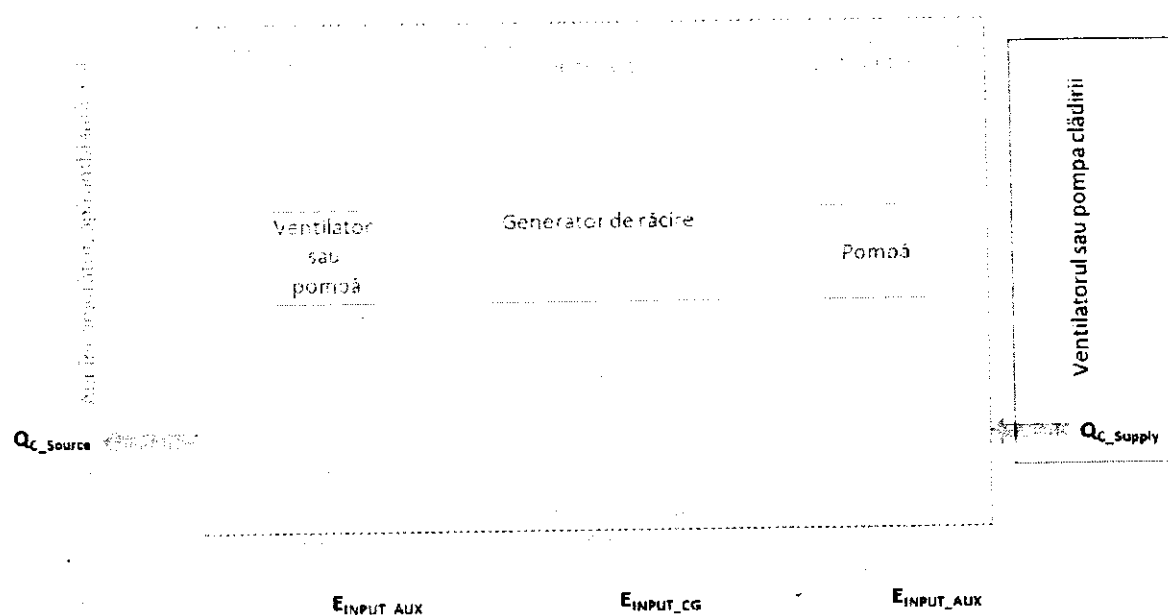
Figura 1 Ilustrarea condițiilor-limită ale FPS pentru generatorul de răcire care utilizează FPS standard și răcirea centralizată (și alte sisteme de răcire de dimensiuni mari care utilizează FPS măsurat), unde E_{INPUT\_AUX} este energia de intrare pentru ventilator și/sau pompă și E_{INPUT\_CG} energia de intrare pentru generatorul de răcire
